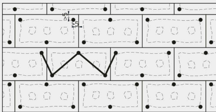
Slika 40. „W-shema“ postavljanja pričvrsnica kod ploča od mineralne vune
