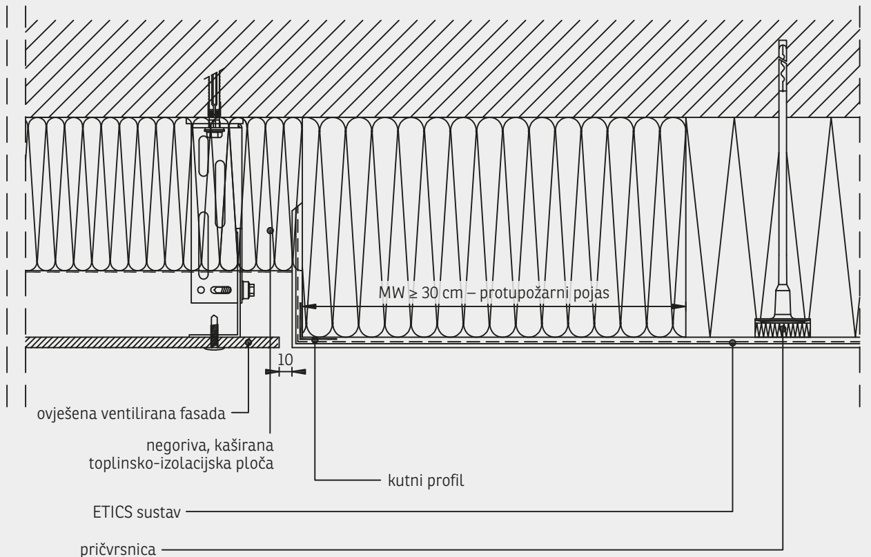
Slika 16. Spoj ETICS-a i ovješnog ventiliranog fasadnog sustava
