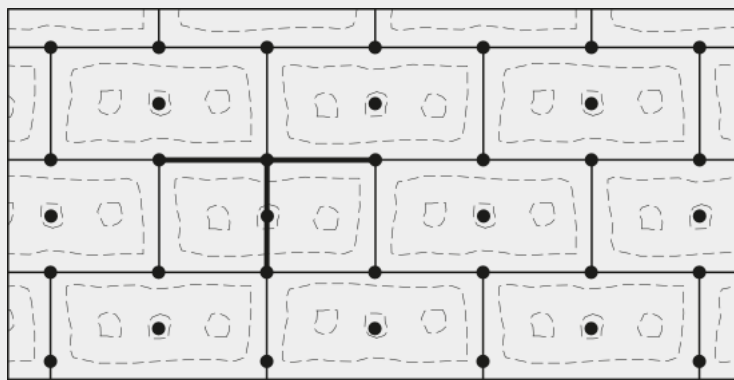
Slika 39. „T-shema“ postavljanja pričvrsnica kod ploča od EPS-a
