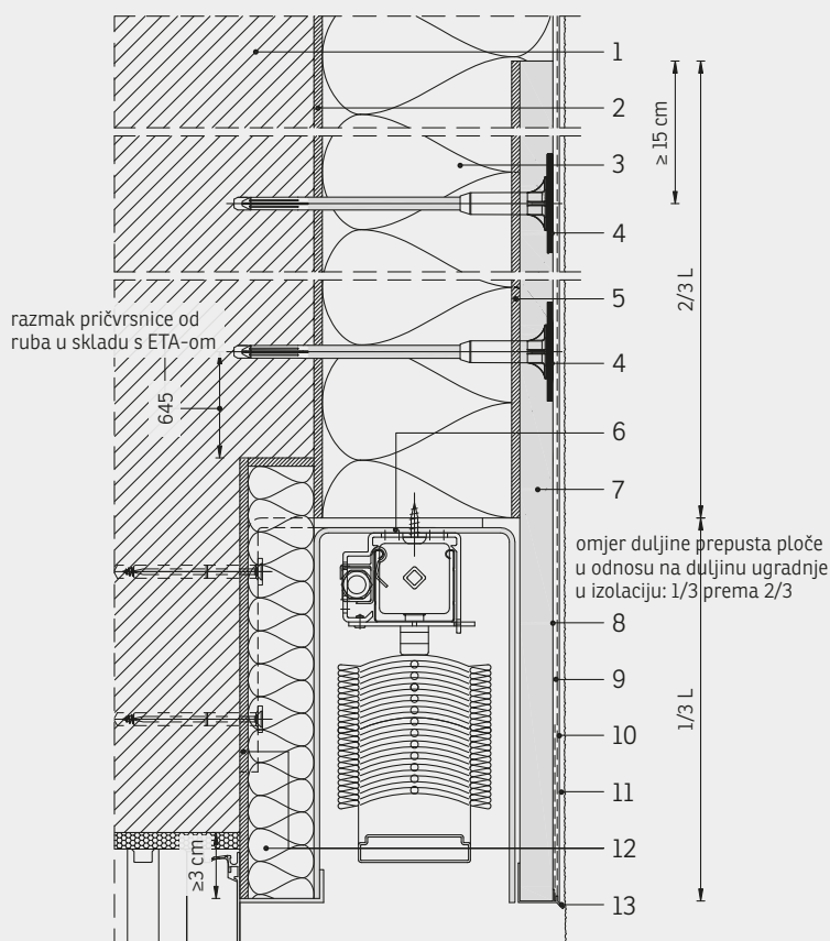
Slika 3. Priključak na nosivu i stabilnu kutiju za rolete bez izolacije na kutiji
