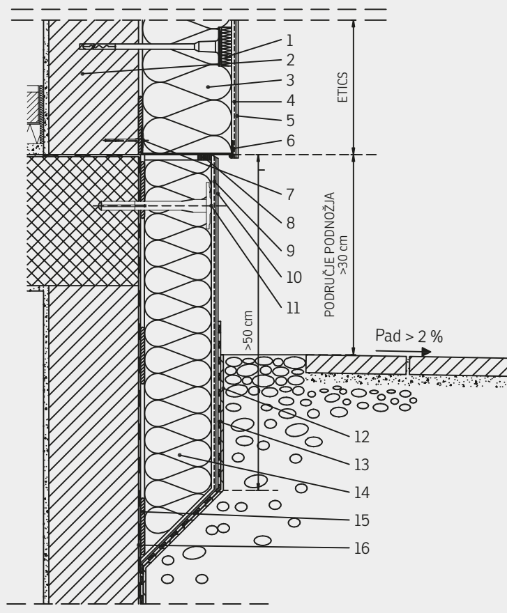
Slika 21. Uvučeno podnožje
