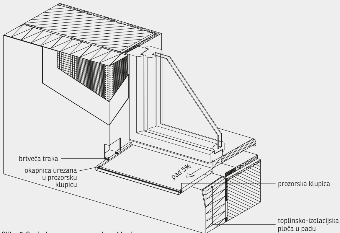
Slika 6. Spoj s kamenom prozorskom klupicom
